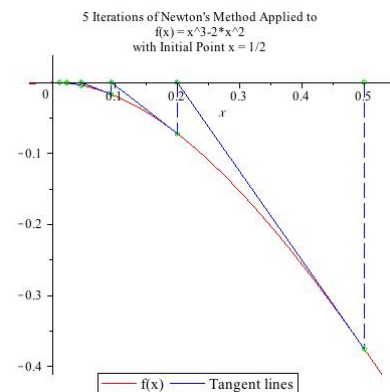
Figura 5.11: Metoda e Njutonit për f(x) = x^3 - 2x^2 .
