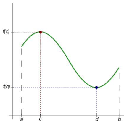
Figura 5.2: Vlerat ekstreme të funksionit
