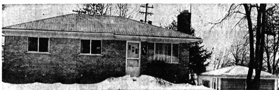
8336 LAGOON
